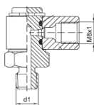
Drehgelenk
