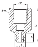
Anschlussstücke mit kegeligem Gewinde
